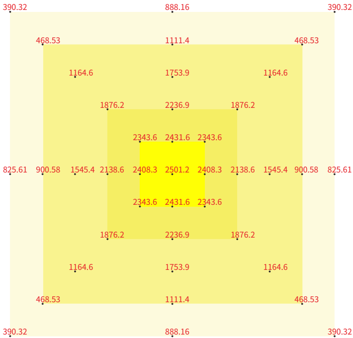
测量高度距灯体30CM, 同平面测量点位间距15CM
