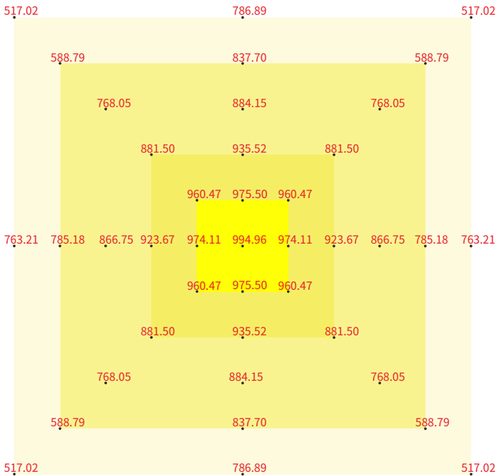
测量高度距灯体100CM, 同平面测量点位间距15CM
