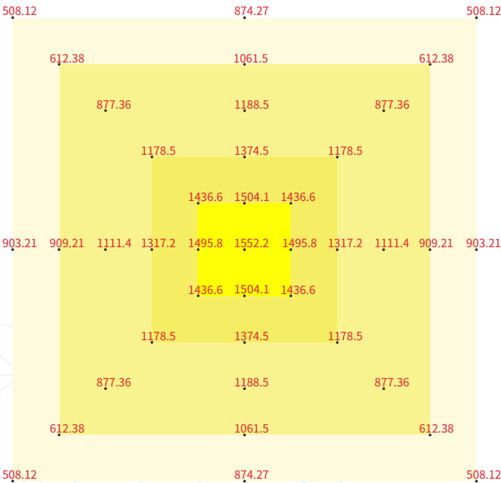
测量高度距灯体60CM, 同平面测量点位间距15CM
