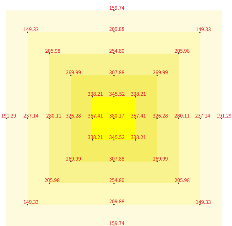
测量高度距灯体60CM,同平面测量点位间距10CM
