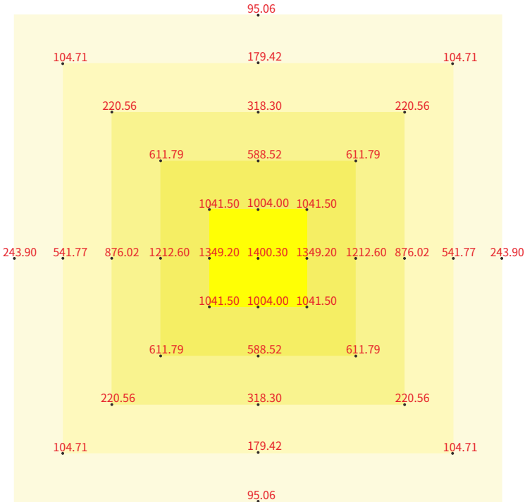
测量高度距灯体30CM,同平面测量点位间距10CM
